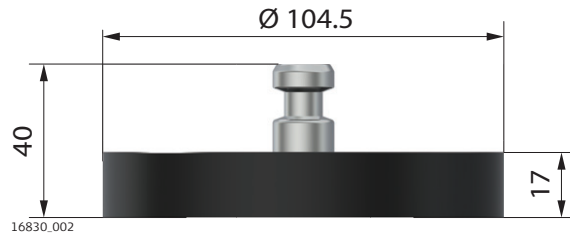
Переходник GAD122 для установки RTC360 на штативе Leica:
