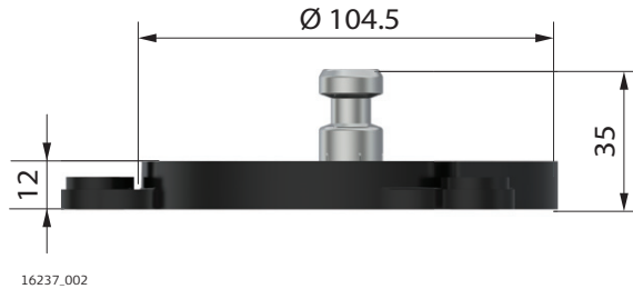
Переходная пластина для гибкого крепления GAD121:
