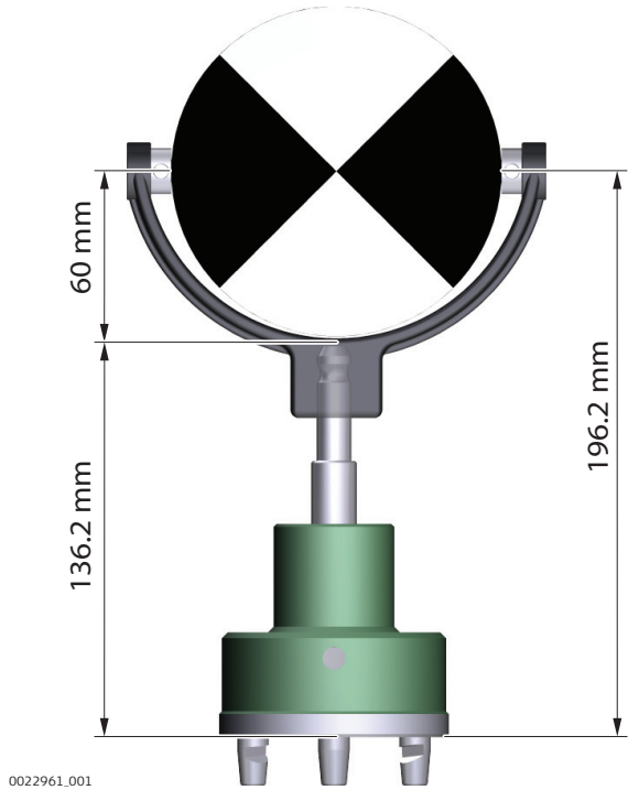
GZT21 Leica Черно-белая мишень 4,5 дюйма на GRT144 адаптере:
